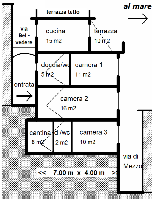
Gebüdeschnitt durch das Haus
